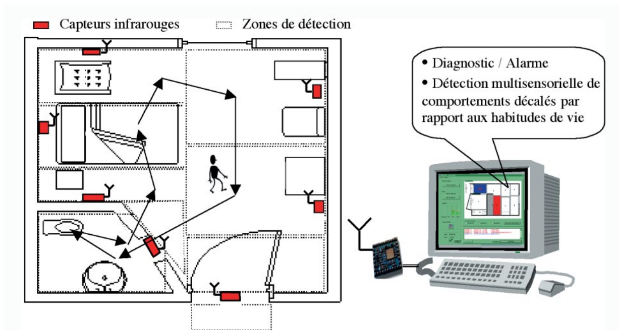
Architecture générale du système PROSAFE version sans fil : les trajectoires de déplacement sont analysées et classifiées pour permettre la détection de toute déviance de trajectoire
