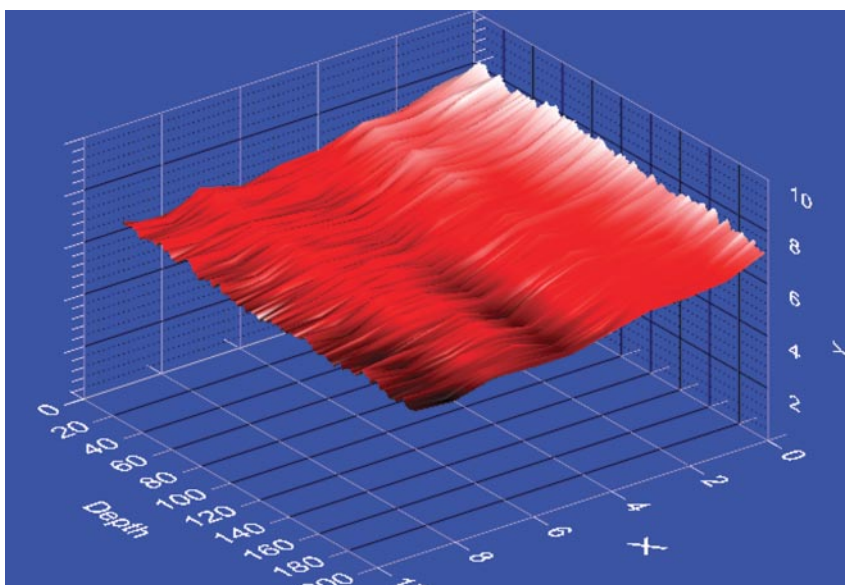
Rendu 3D d'une gravure par RIE
